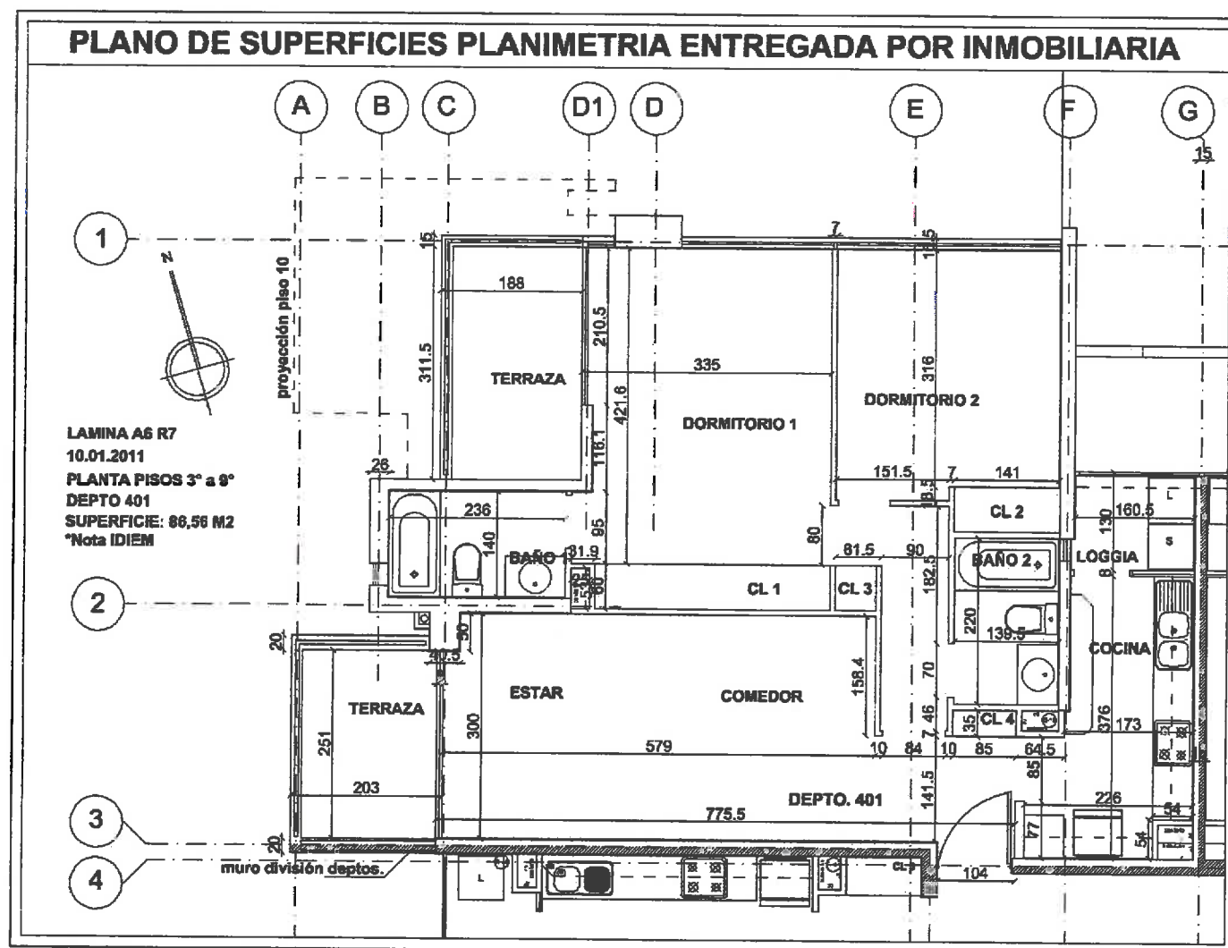
Plano N° 1 Planta de Arquitectura A6 tipo 3° al 9° piso, revisión 7 del 10/01/2011.
