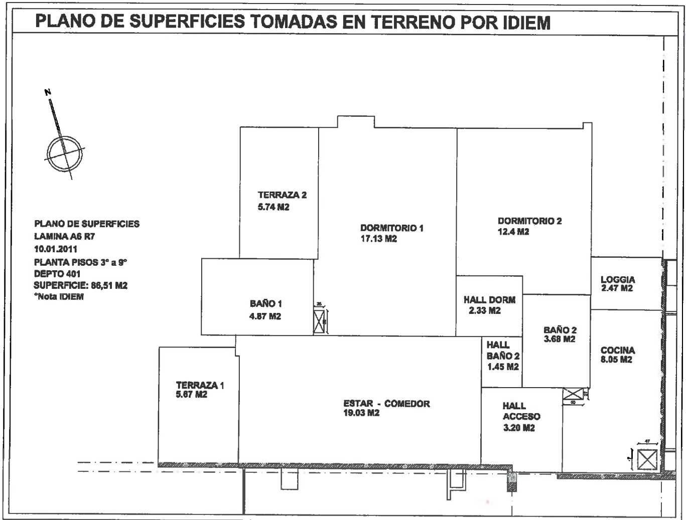
Plano N° 4 con polígonos con superficies de los recintos según medición en terreno IDIEM
