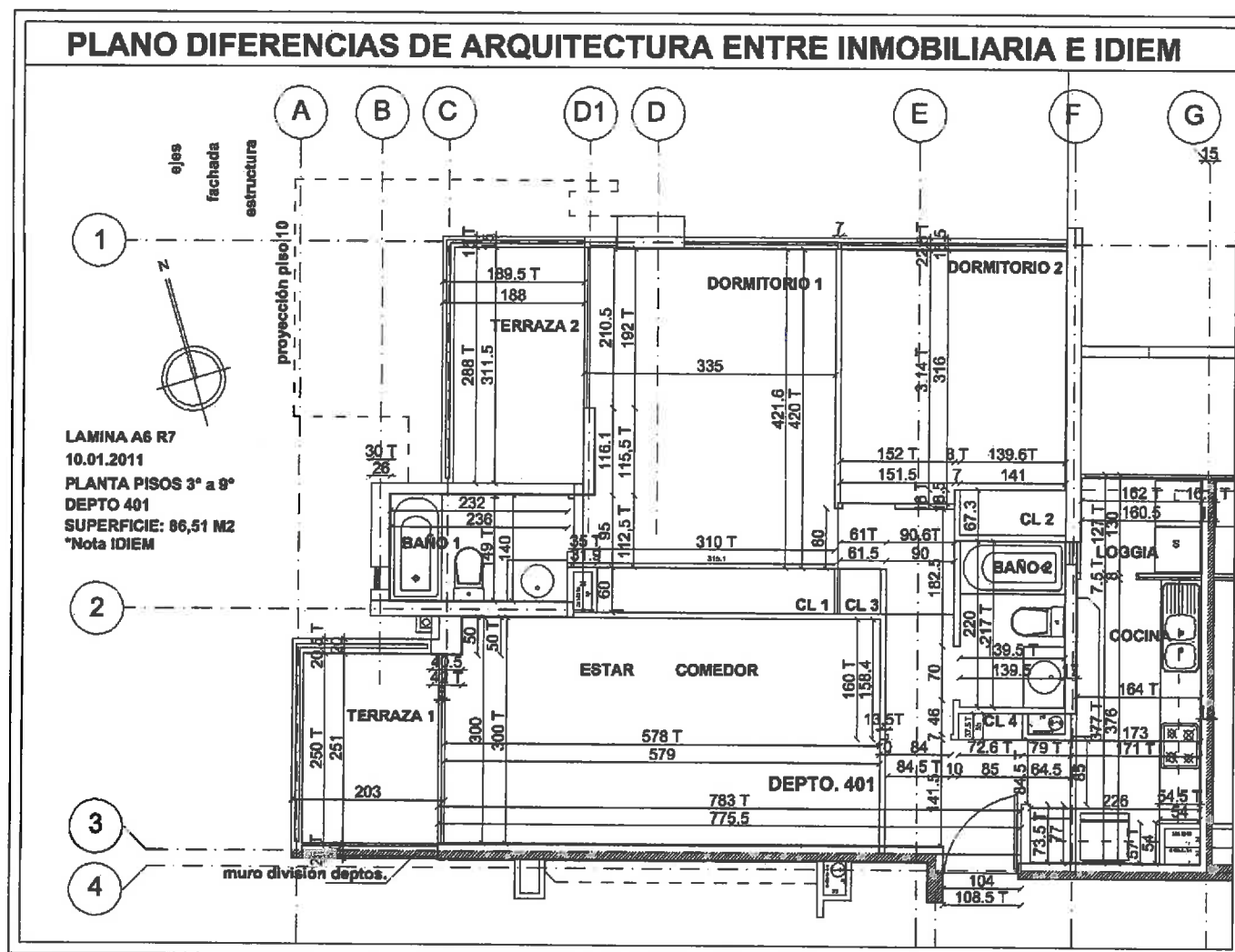
Plano N° 3 con mediciones en Autocad y en terreno.
