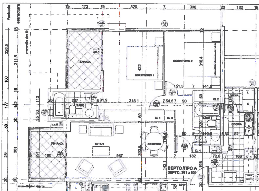
Plano N° 1 Planta de Arquitectura A6 tipo 3° al 9° piso, revisión 7 del 10/01/2011.
