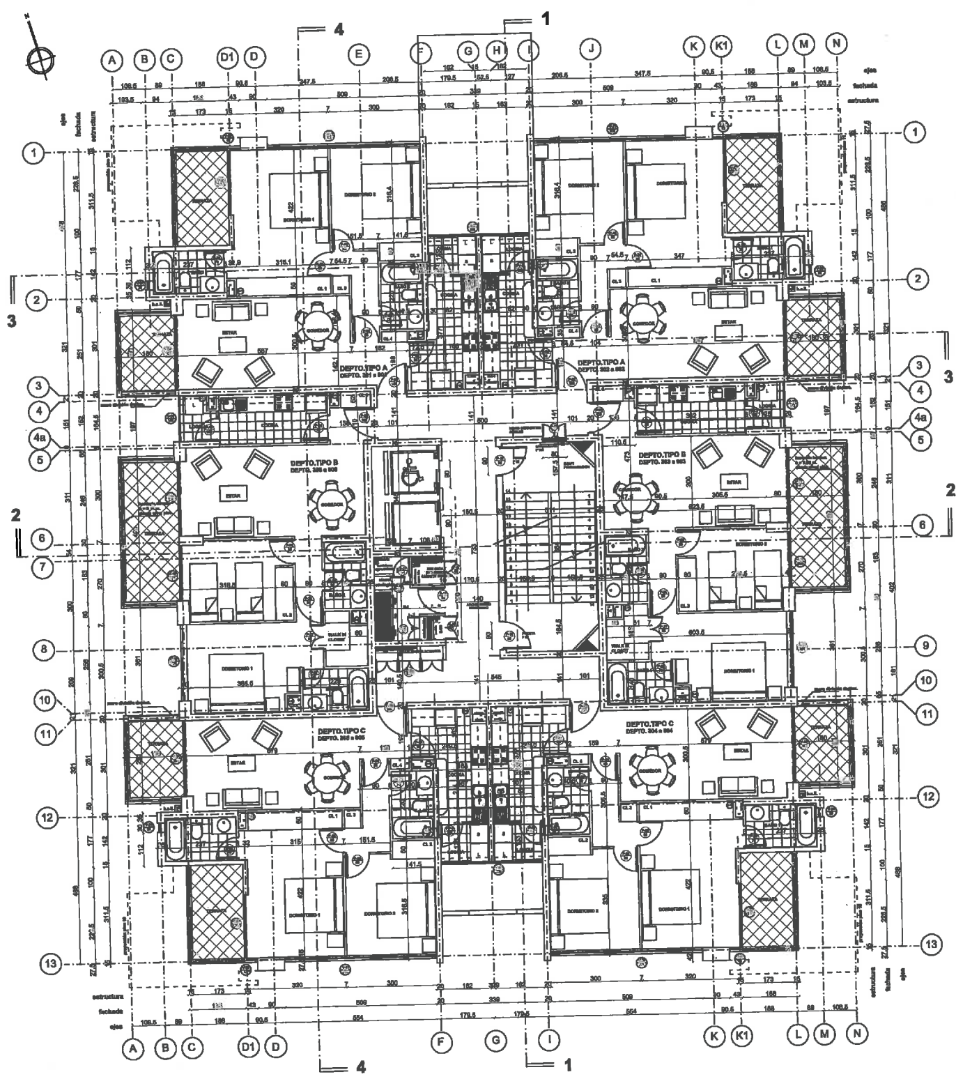
PLANTA PISO TIPO 3° a 9° PISO niveles +5,18 a +20,18 ESCALA 1:50
